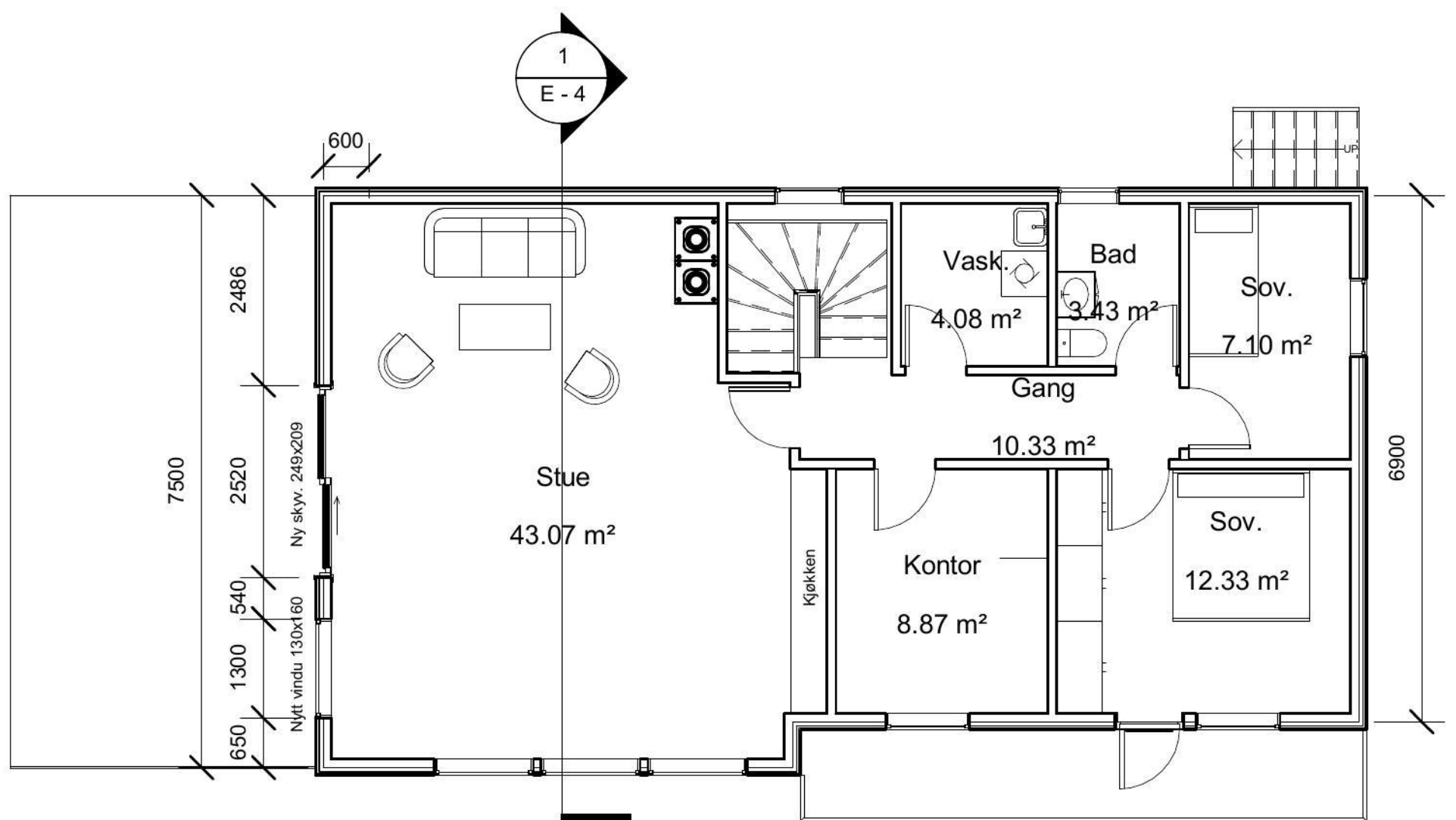
Plan 1 etg.
